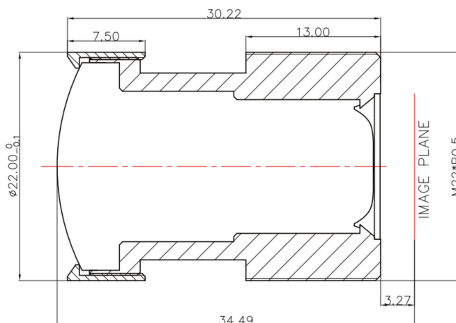
尺寸示意图
