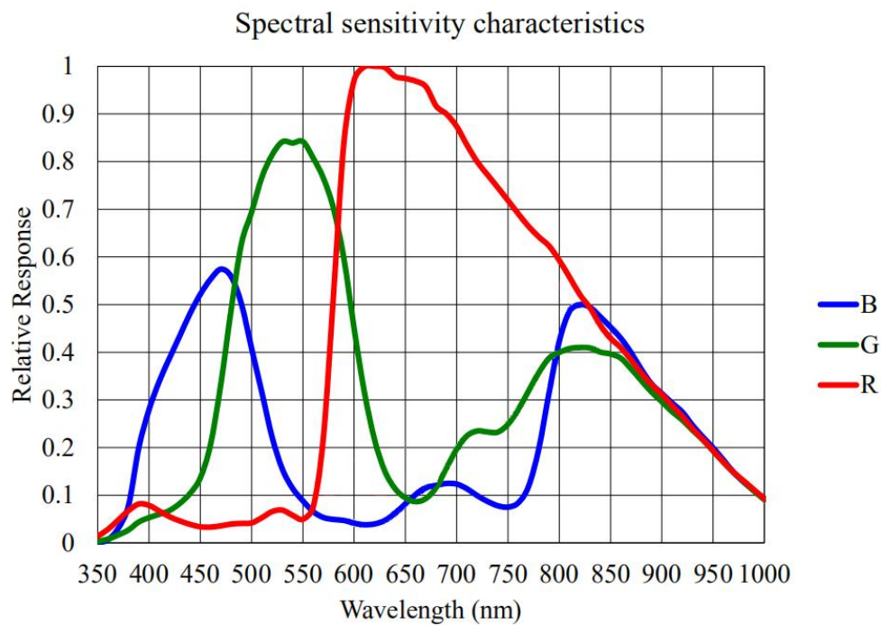
JHUM806s 波谱响应图
