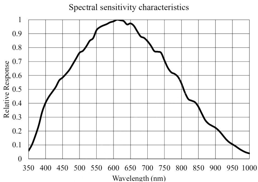
JHUM806Bs 波谱响应图
