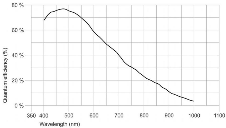
JHUM600Bs 波谱响应图
