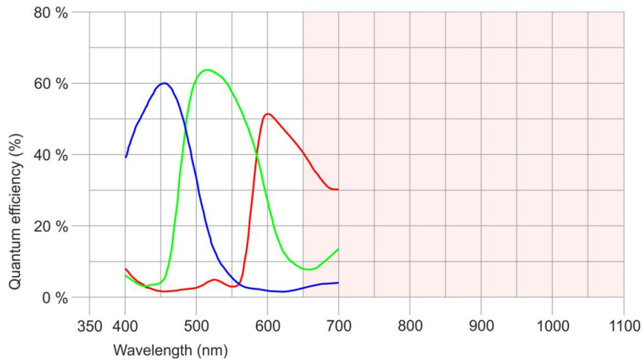
JHUM600s 波谱响应图
