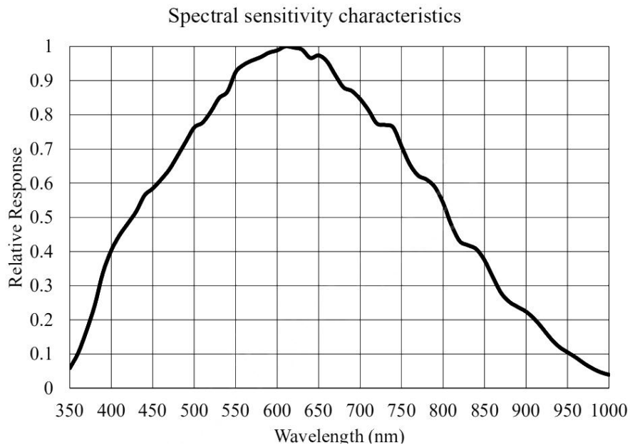
JHUM506Bs 波谱响应图
