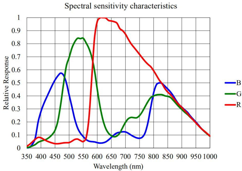
JHUM506s 波谱响应图
