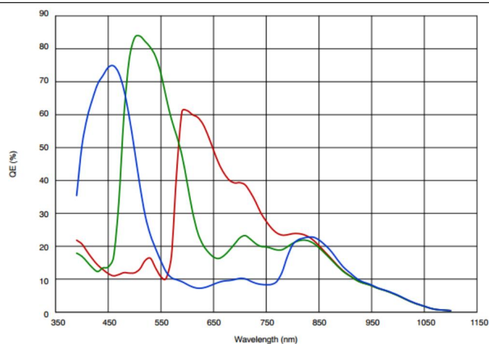
图一： 芯片波谱响应图
