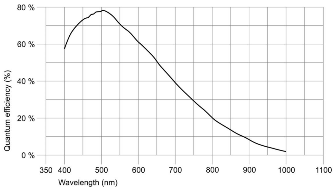
JHUM214Bs 波谱响应图
