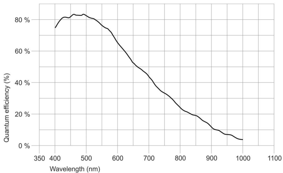
JHUM2000Bs 波谱响应图
