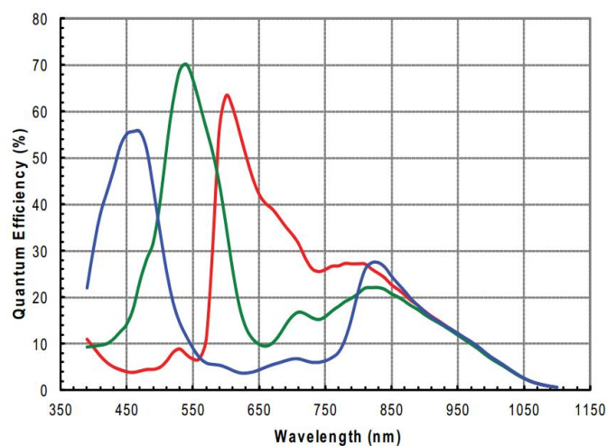
图一： 芯片波谱响应图
