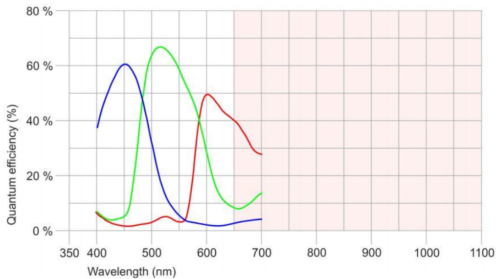
JHUM1200s 波谱响应图
