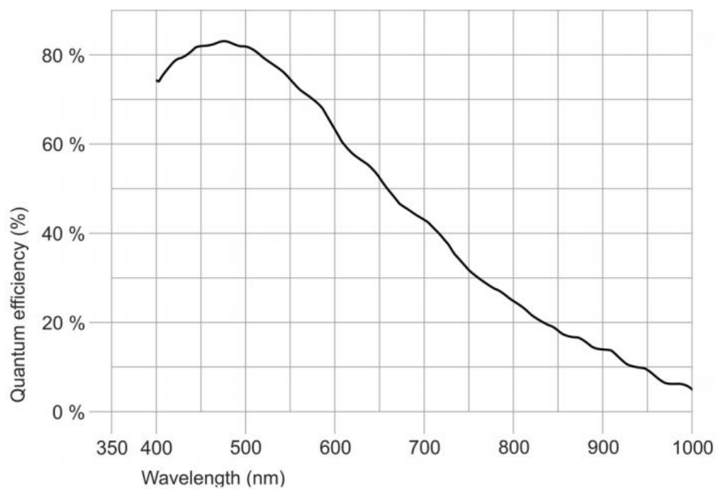
JHUM1200Bs 波谱响应图
