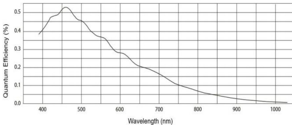
图一： 芯片波谱响应图
