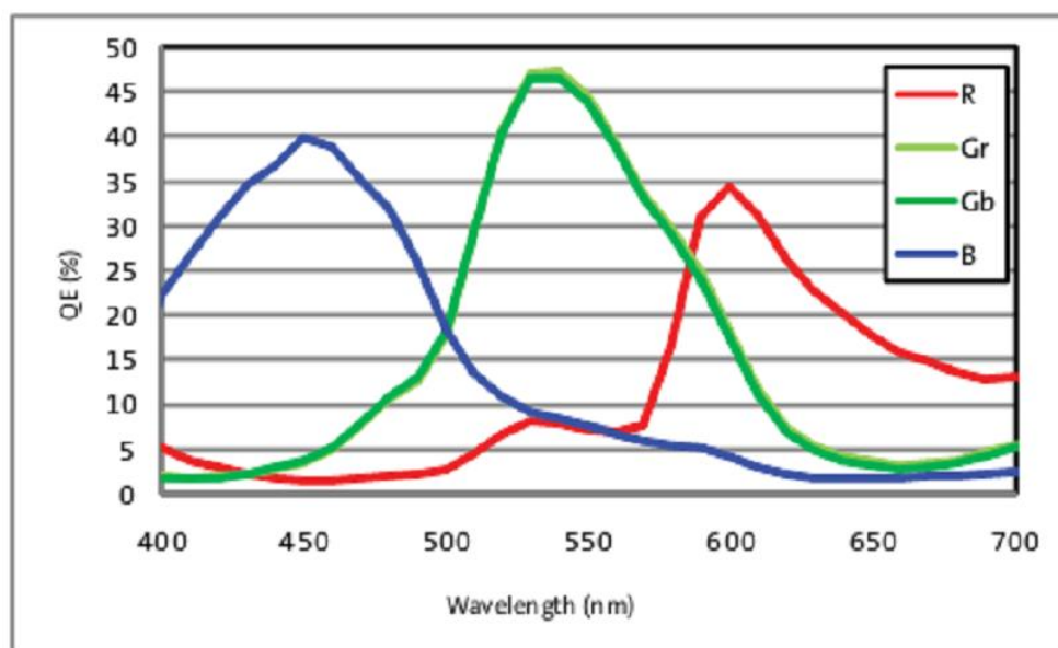
图 1 光谱响应图
