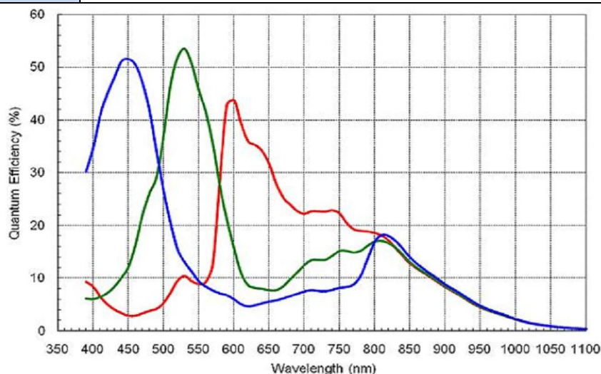
图一： 芯片波谱响应图
