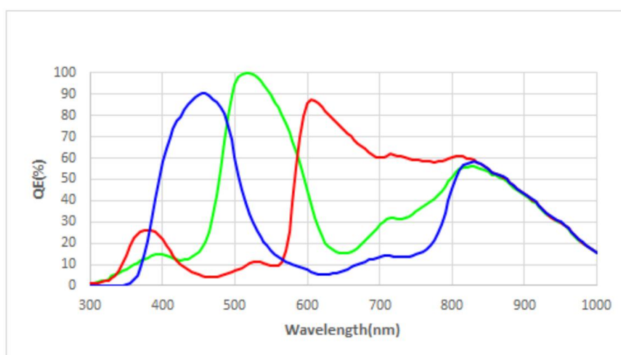
图一： 芯片波谱响应图
