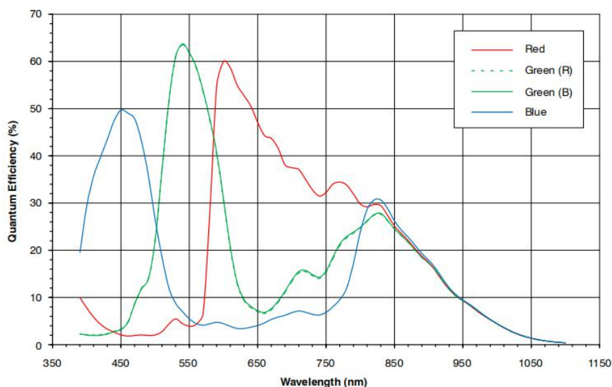
图一： 芯片波谱响应图
