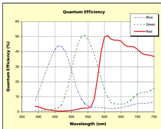
图一： 芯片波谱响应图
