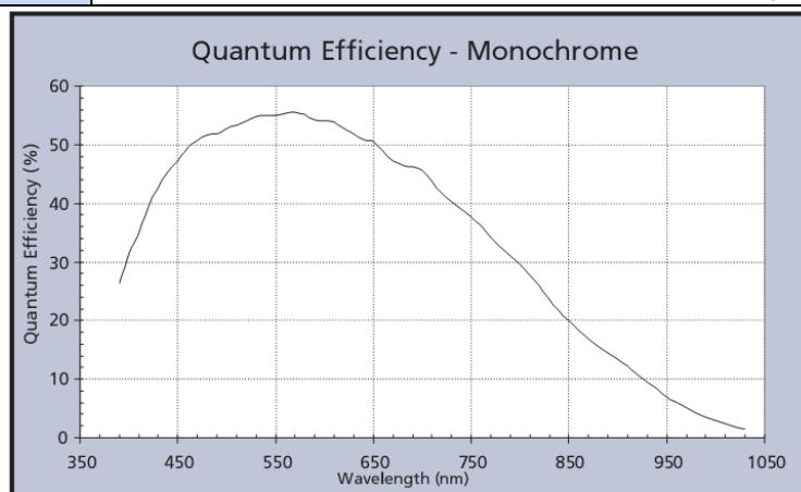
图一： 芯片波谱响应图
