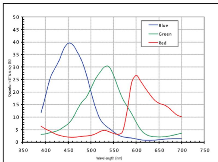
图一： 芯片波谱响应图
