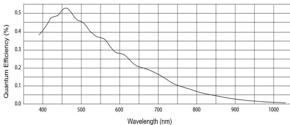
图一： 芯片波谱响应图
