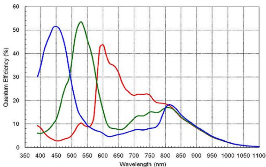
图 1 光谱响应图
