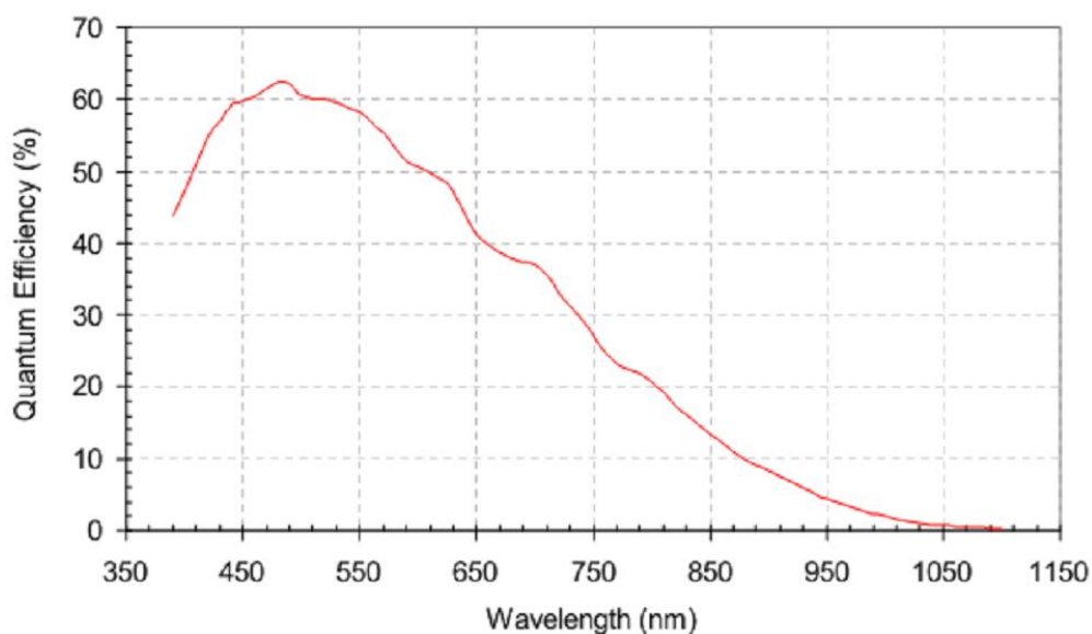
图 1 光谱响应图
