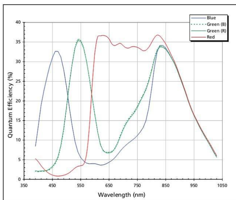
图 1 光谱响应图
