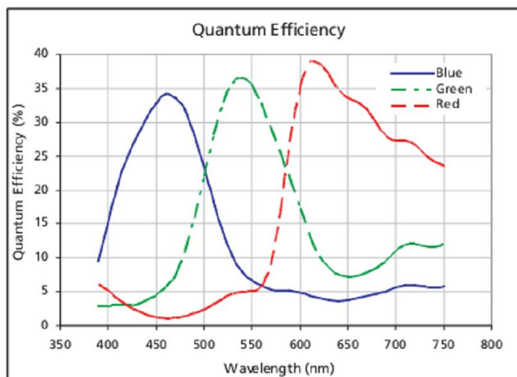
图 1 光谱响应图
