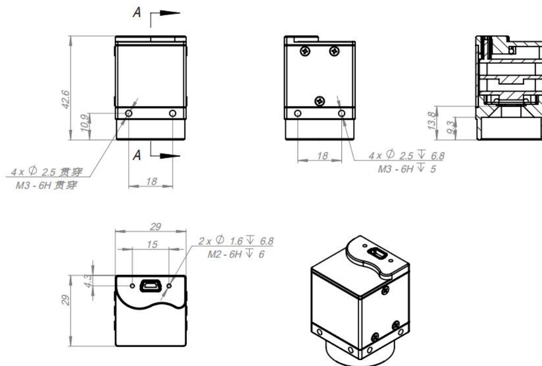
安装尺寸图 (单位: mm)
