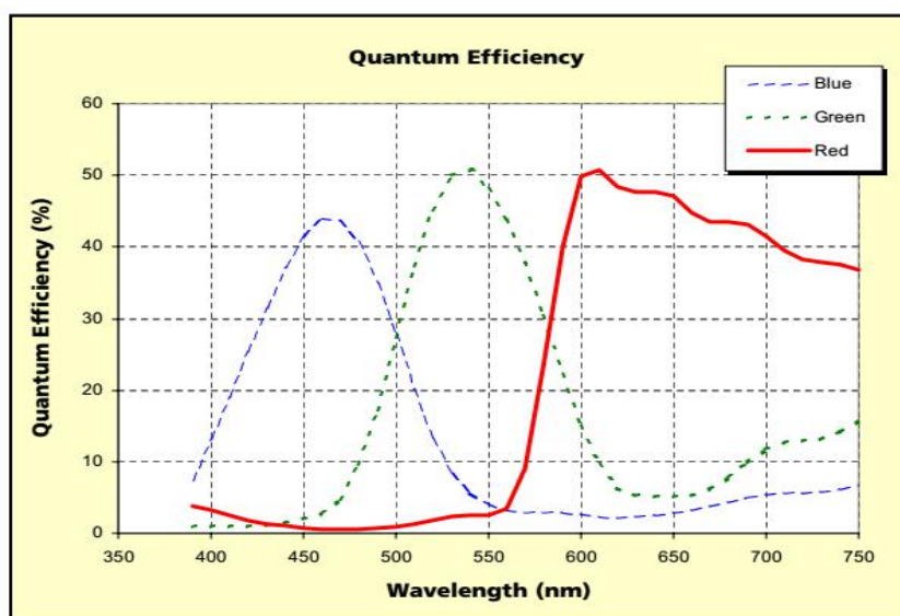
图 1 光谱响应图
