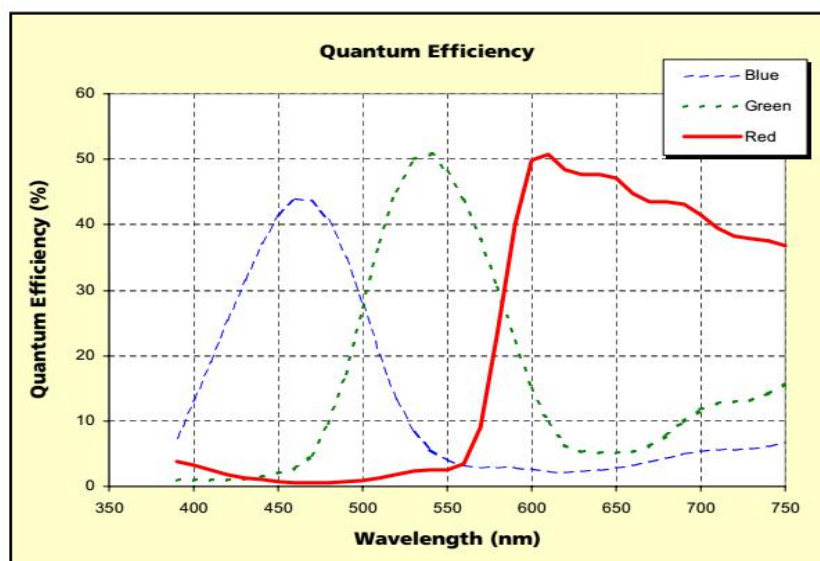
图 1 光谱响应图
