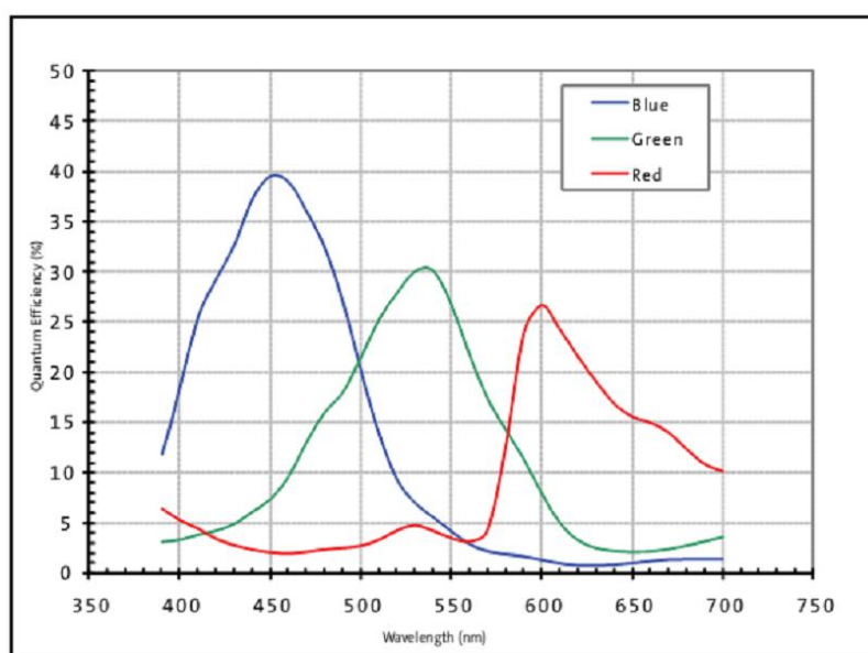
图 1 光谱响应图
