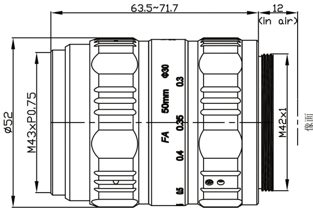
尺寸示意图
