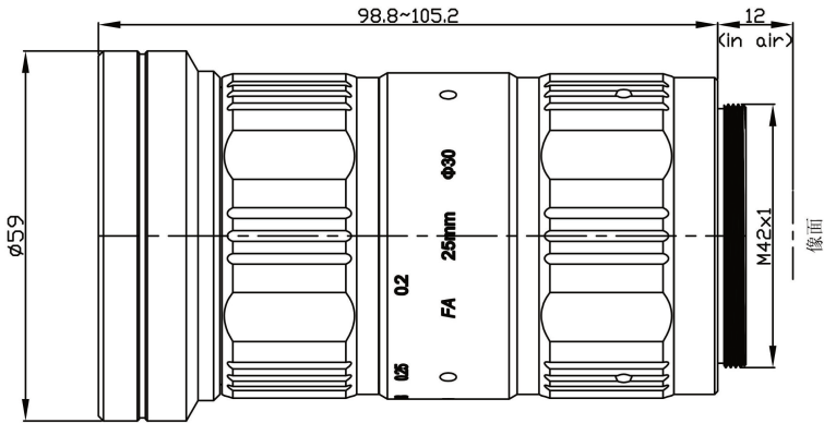
尺寸示意图
