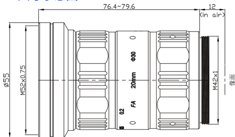
尺寸示意图
