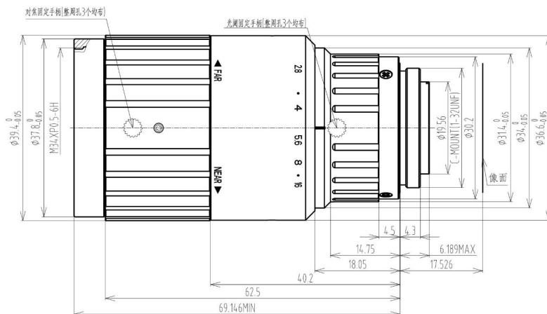
尺寸示意图
