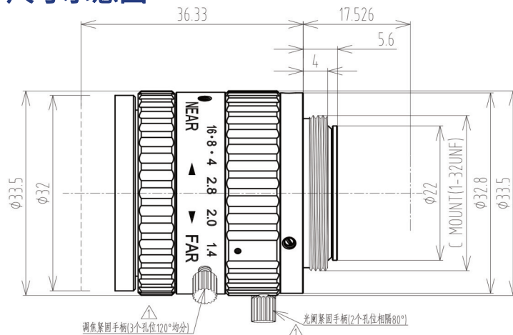
尺寸示意图
